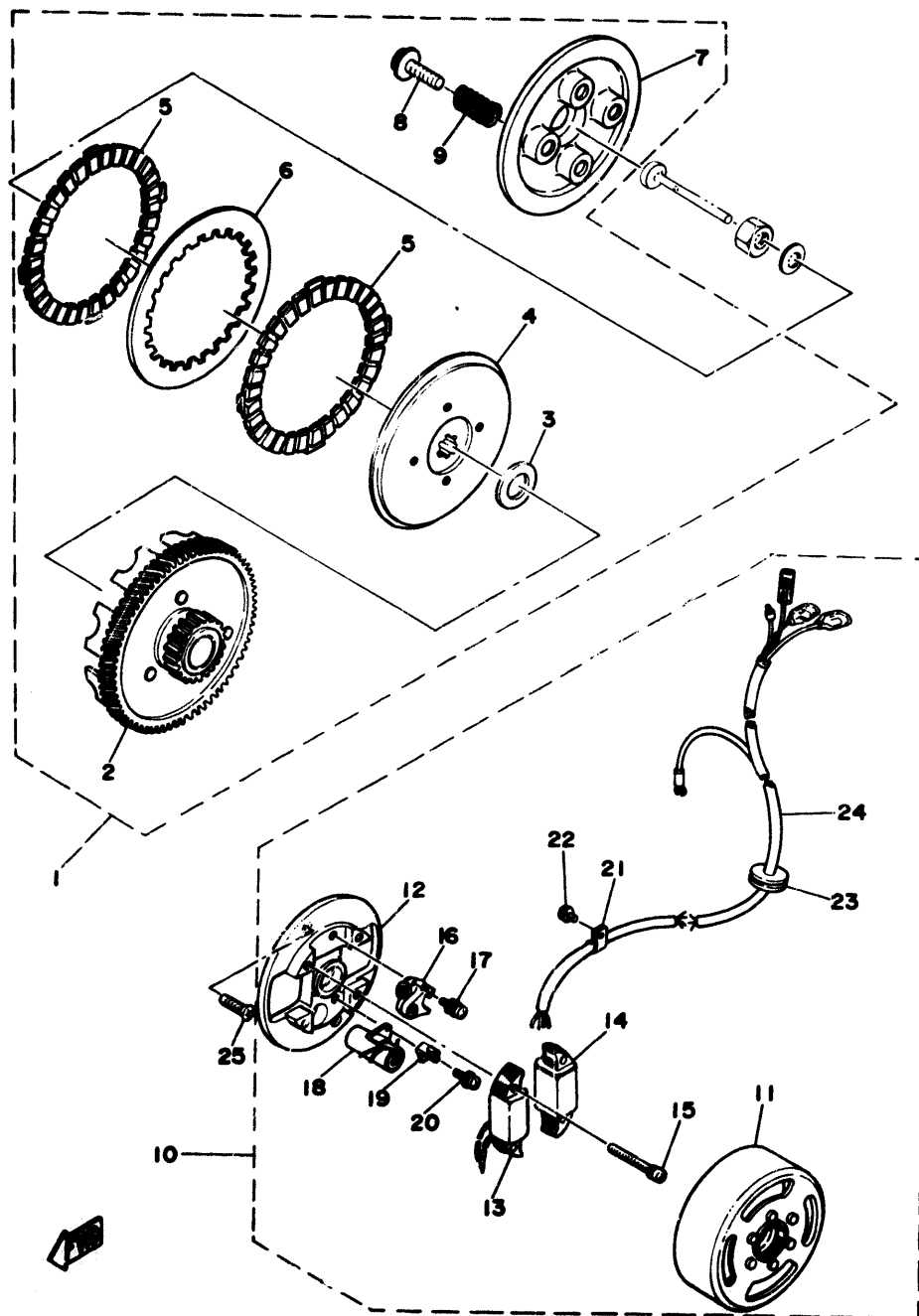
Fig. 1 CLUTCH · FLYWHEEL MAGNETO
