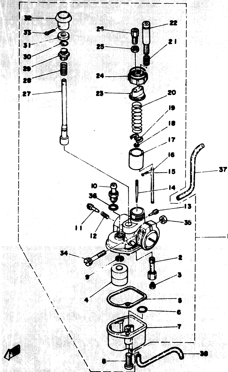
Fig. 10 CARBURETOR
