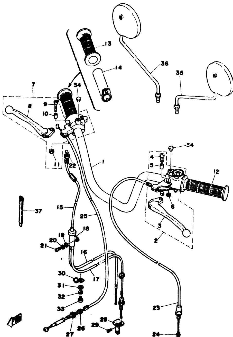
Fig. 22 HANDLE · WIRE (FS1)
