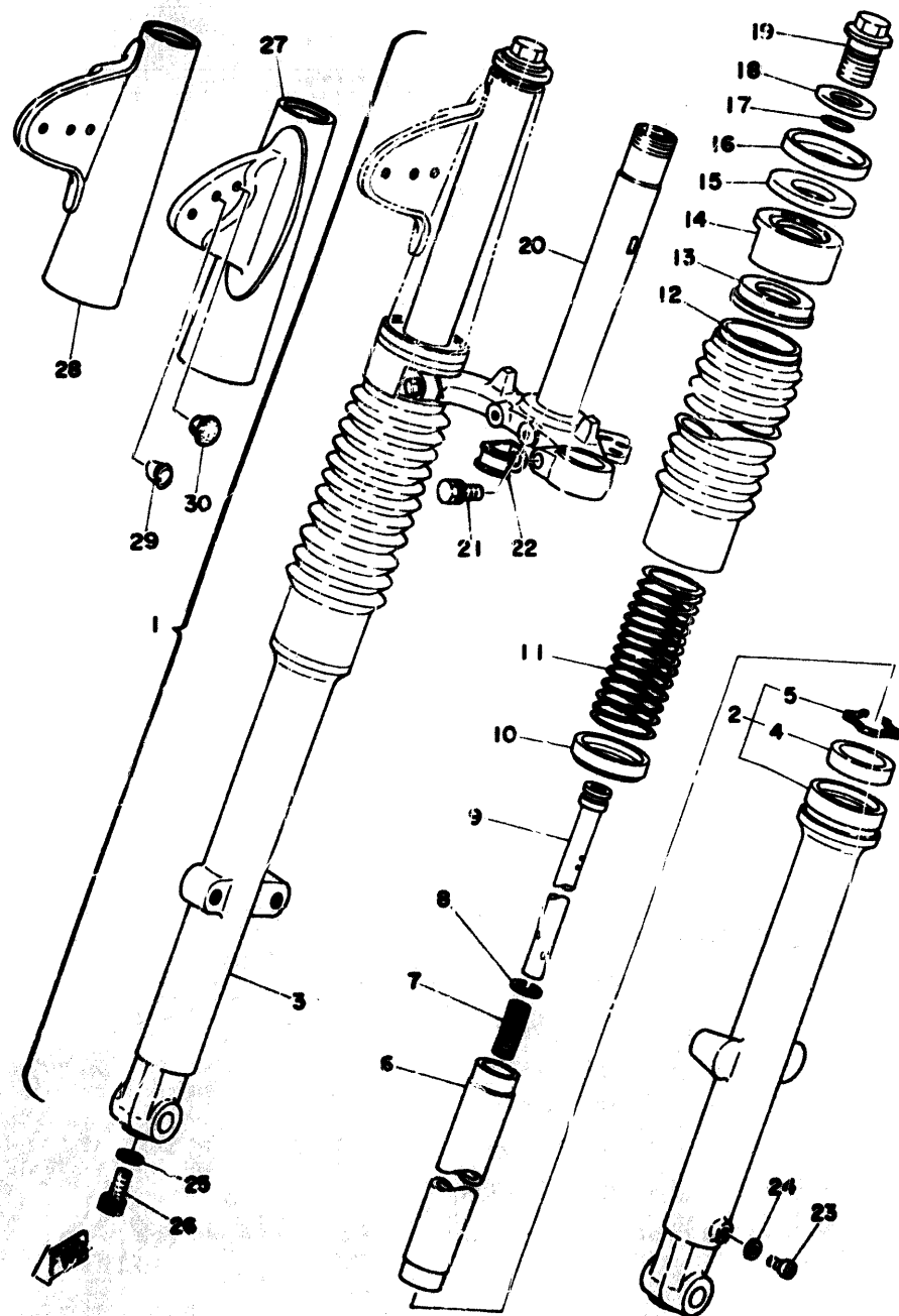
Fig. 20 FRONT FORK (FS1-DX)
