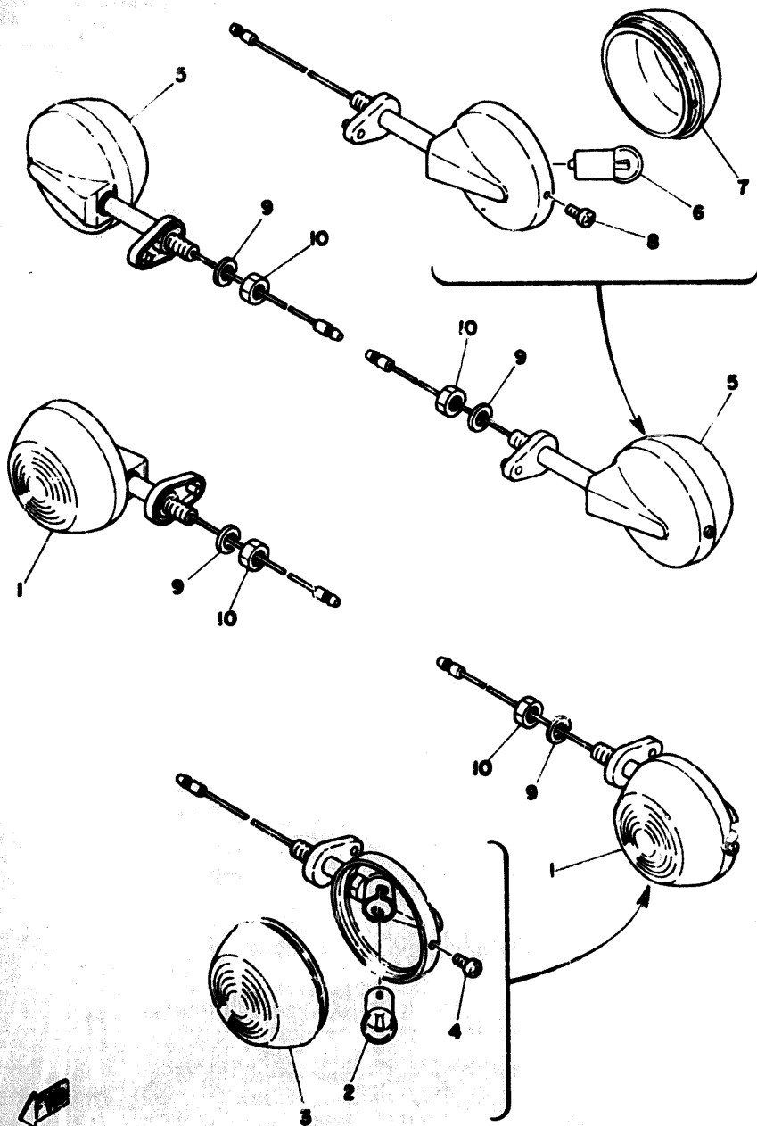
Fig. 38 FLASHER LAMP 2
