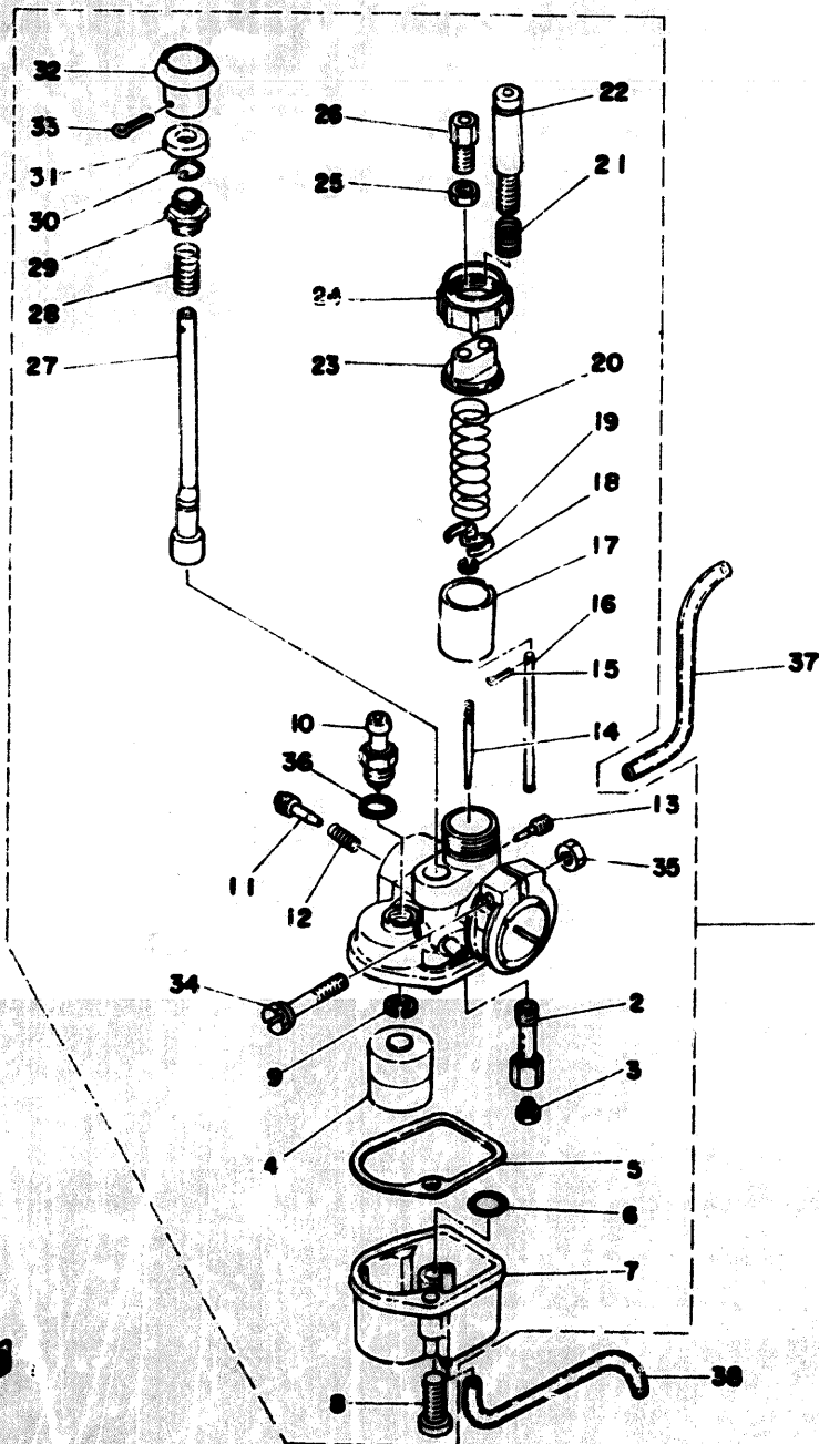
Fig. 10 CARBURETOR
