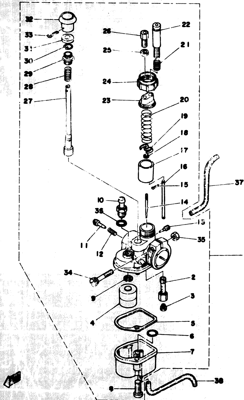
Fig. 10 CARBURETOR
