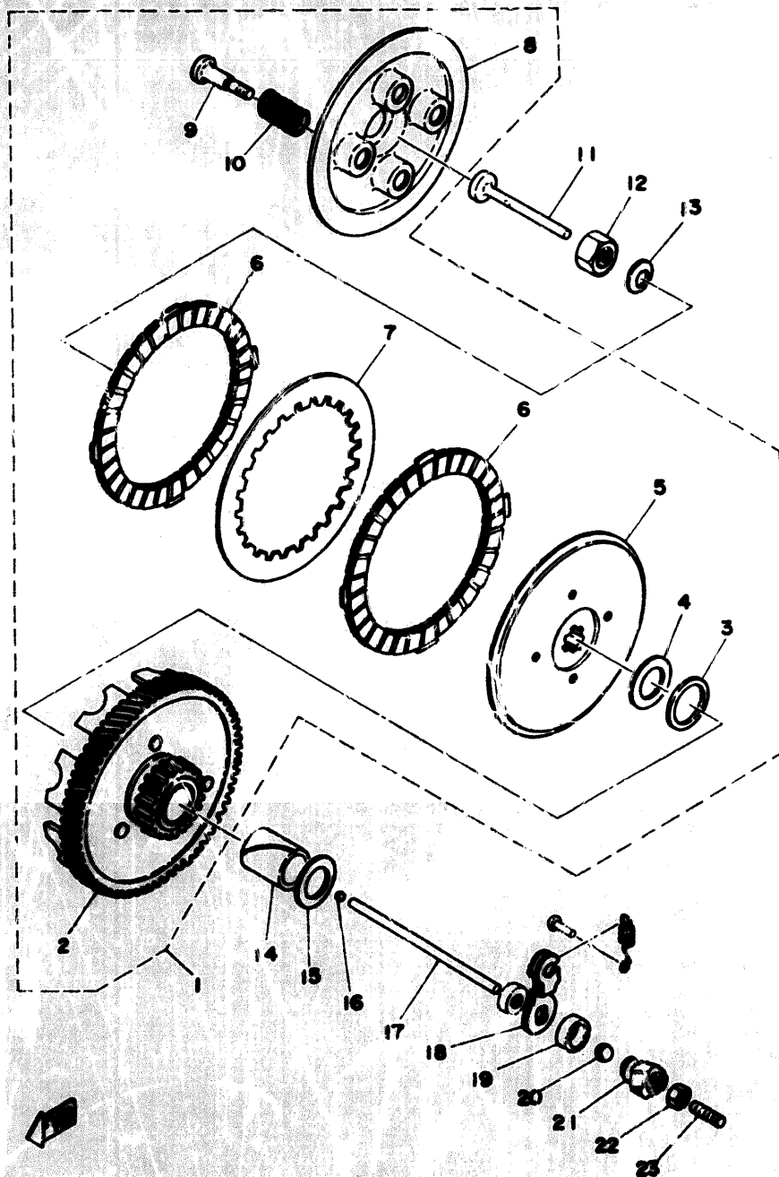
Fig. 4 CLUTCH
