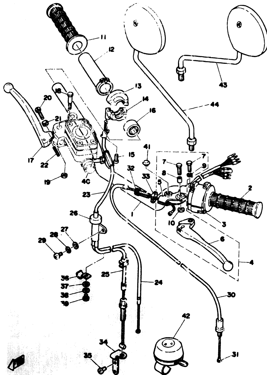
Fig. 23 HANDLE · WIRE (FS1-DX)
