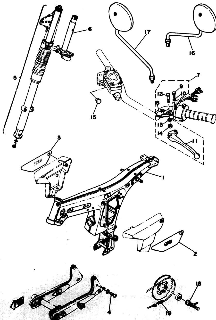
Fig. 2 FRAME · FRONT FORK · HANDLE
