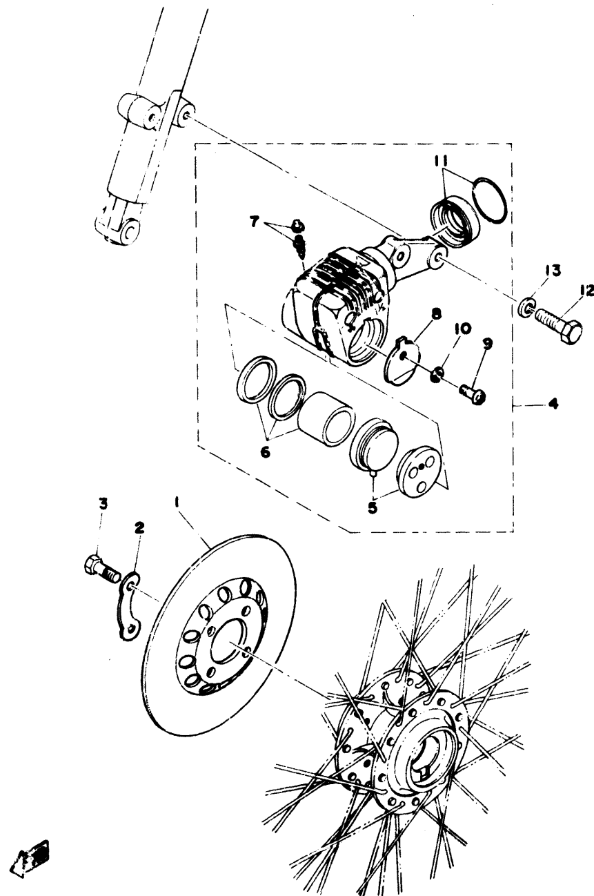
Fig. 30 DISC BRAKE · CALIPER (FS1-DX)
